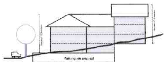
Hypothèse 1 - coupe de principe
